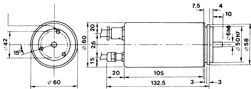
TKC 260 flangia "H" TKC 260 "H" flange
